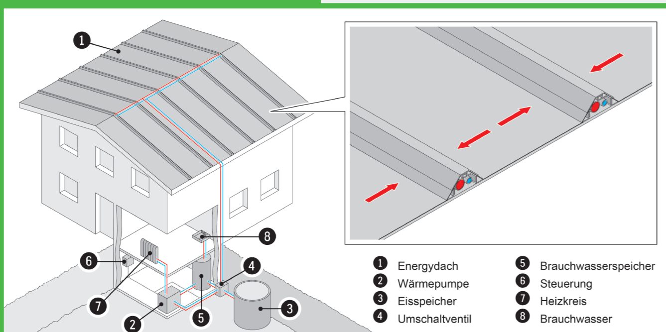
Gesamtsystem mit Wärmepumpe und Eisspeicher
